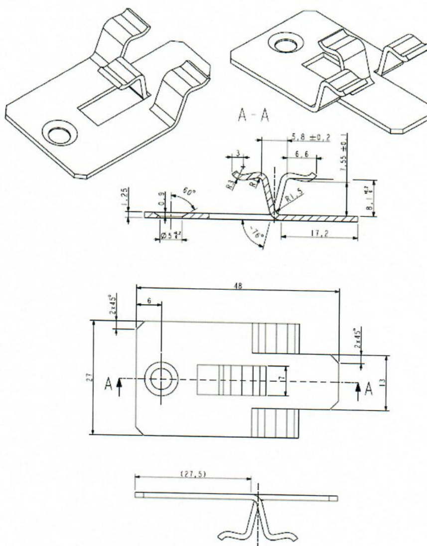
Rysunek A4. Klips montażowy
