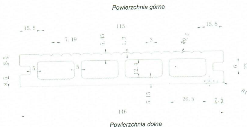
Rysunek A2. Deski tarasowe o wymiarach przekroju 146 x 23 mm, ryflowane jednostronnie
