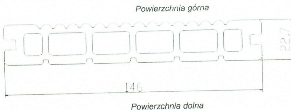
Rysunek A1. Deski tarasowe o wymiarach przekroju 146 x 22,7 mm, ryflowane obustronnie
